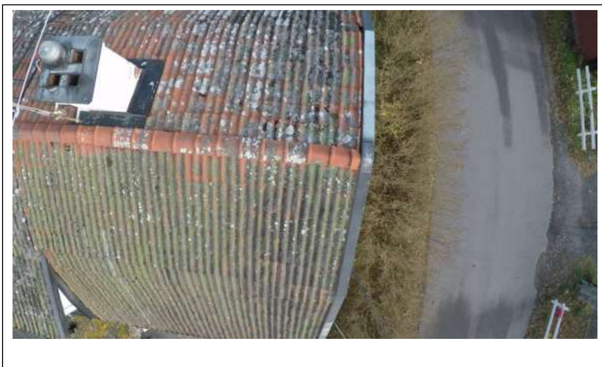
Figur 2, putssläpp noterades vid murad skorsten.
